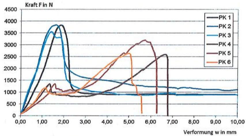
Bild 1: Last-Verformungskurven
